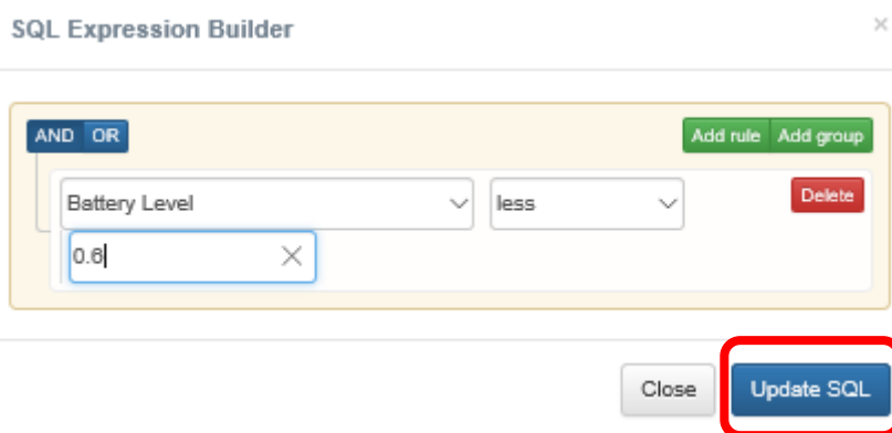
Slika 12. SQL Expression Builder
